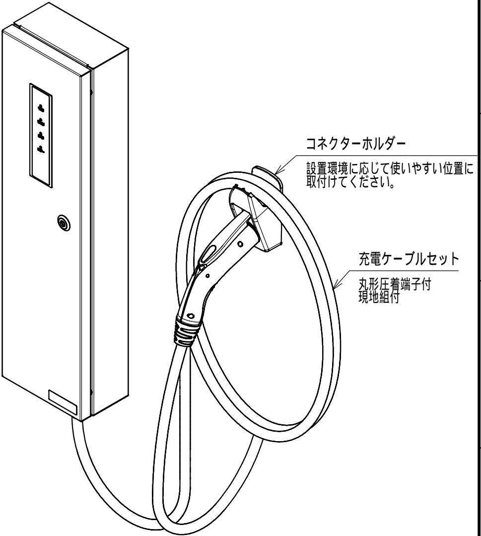
<取付例> 壁面取付
