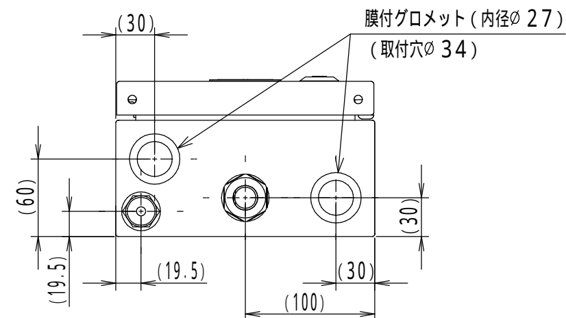
底面詳細図 (1:4)
