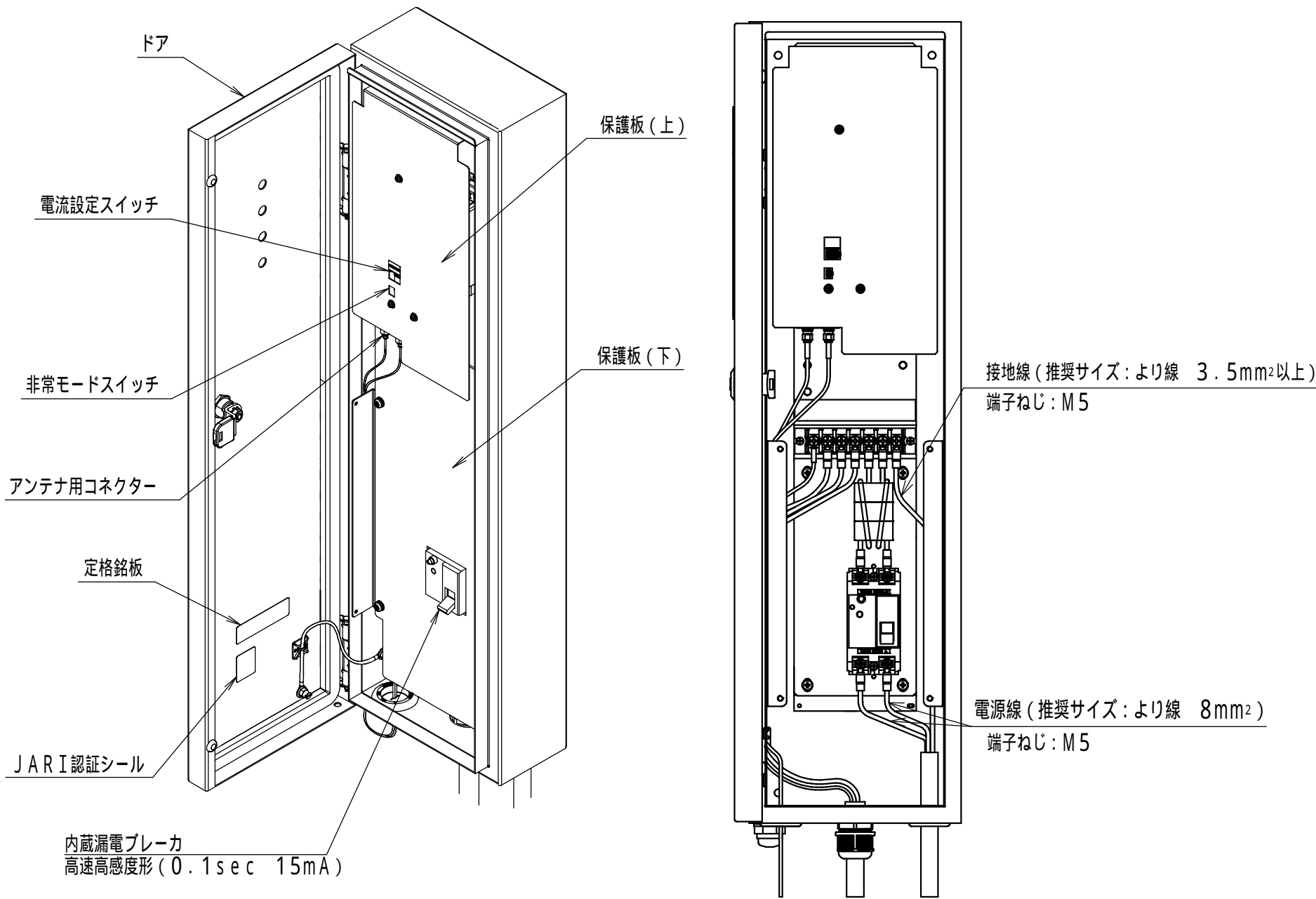
充電器内面図 ドアを開けた図
