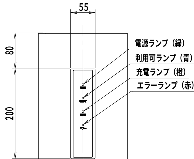
インフォメーションパネル詳細図 (1:5)
