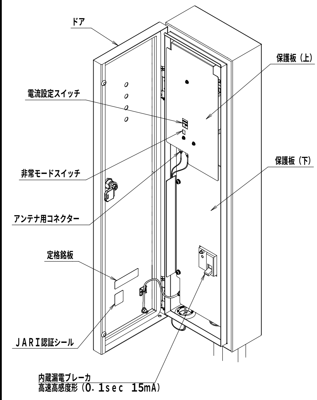
充電器内面図 ドアを開けた図
