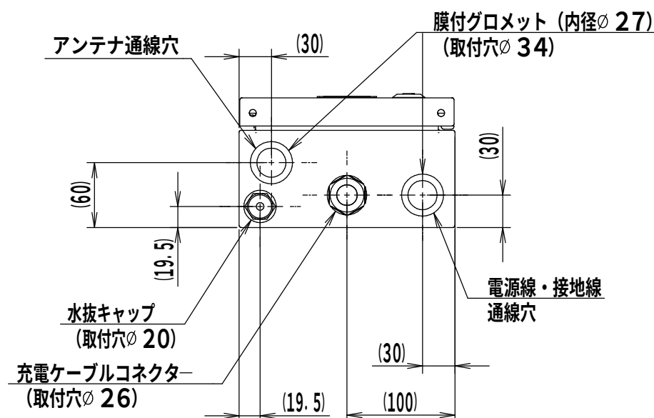
充電器本体の底面詳細図 (1:5)
