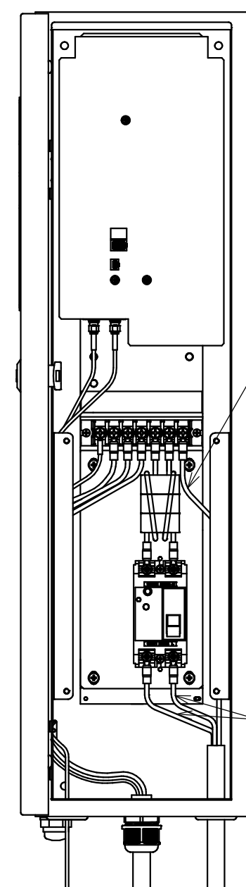
充電器内部配線図 (1:5) 保護板 (下) を外した図
