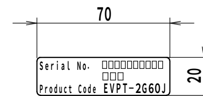
シリアルラベル詳細図 (1:2)
