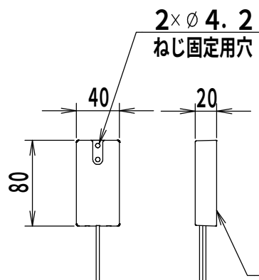
アンテナ詳細図 (1:5)
