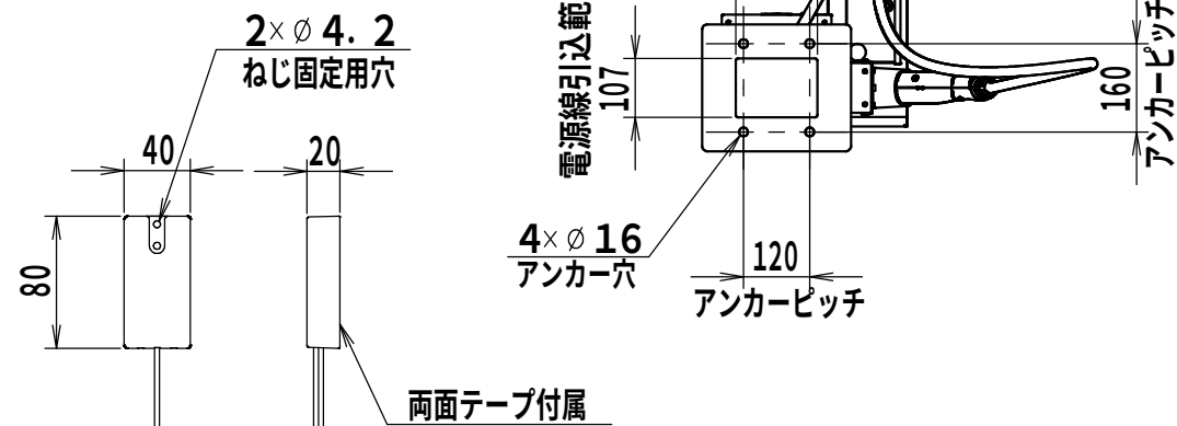
アンテナ詳細図 (1:5)
