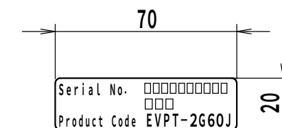
シリアルラベル詳細図 (1:2)
