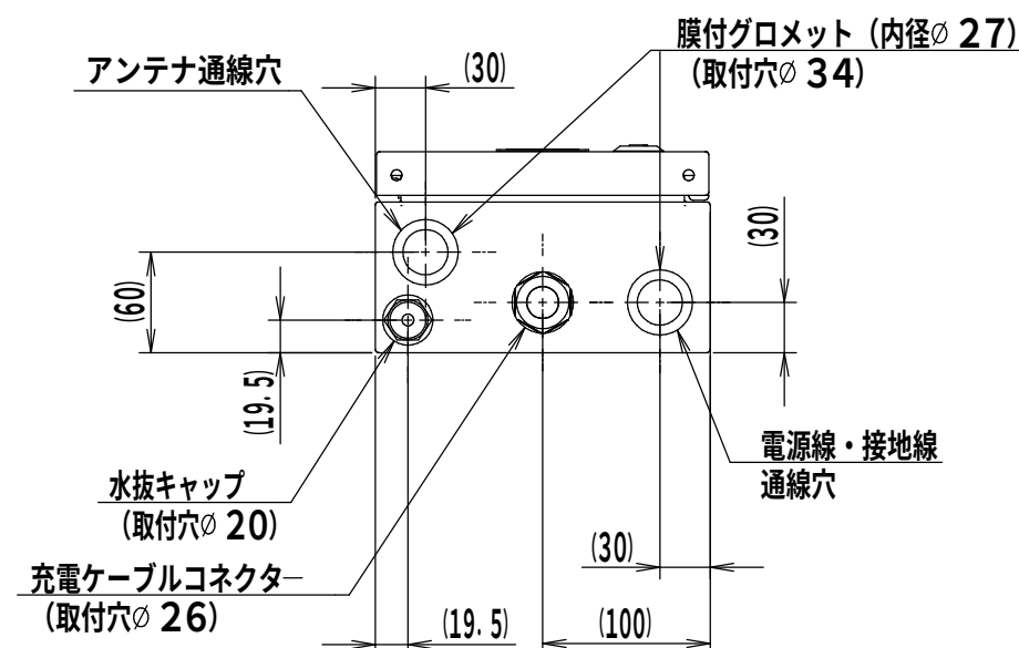
インフォメーションパネル詳細図 (1:5)
