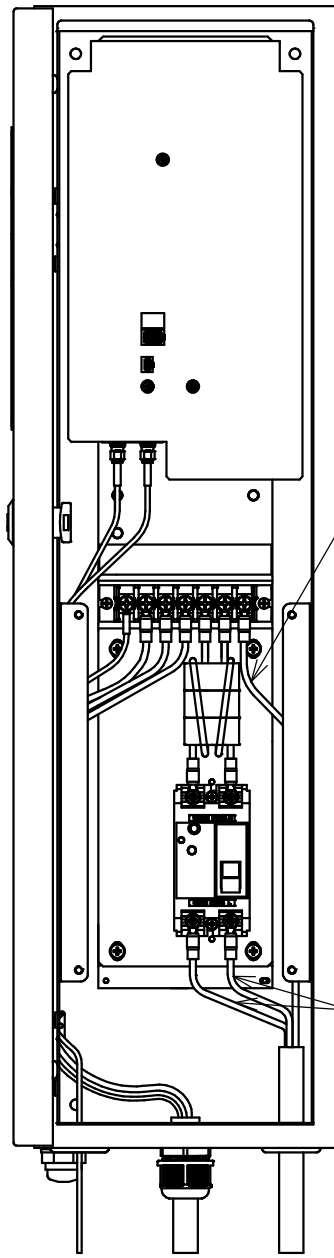
充電器内部配線図 (1:5) 保護板 (下) を外した図
