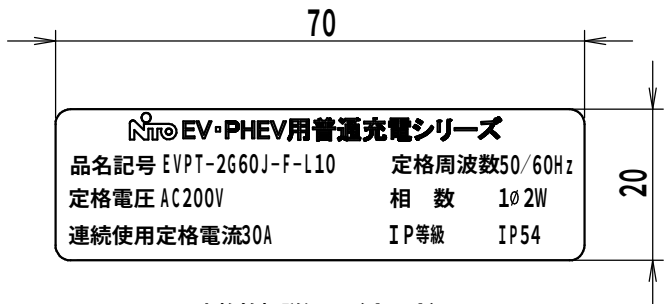
定格銘板詳細図 (1:1) (ドア裏貼付)
