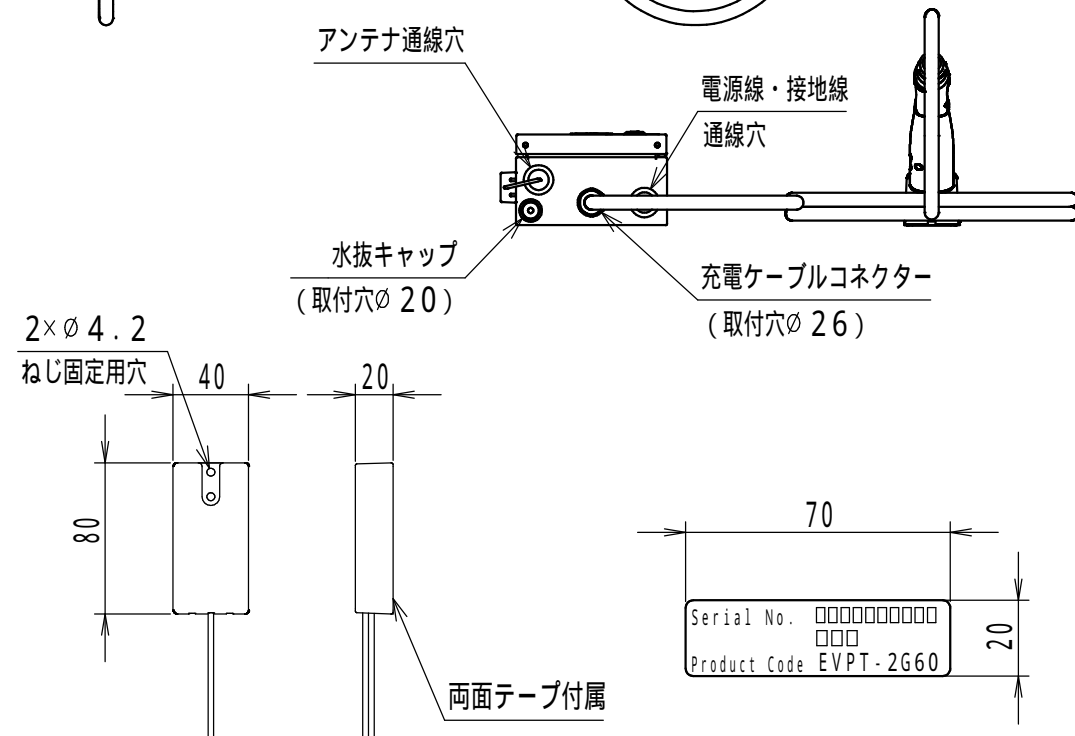
アンテナ詳細図 (1:4)
