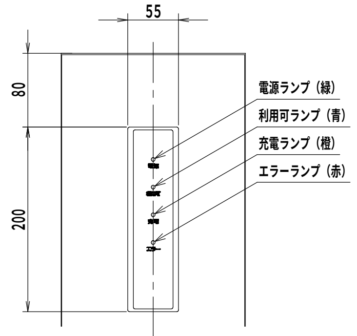
インフォメーションパネル詳細図 (1:4)
