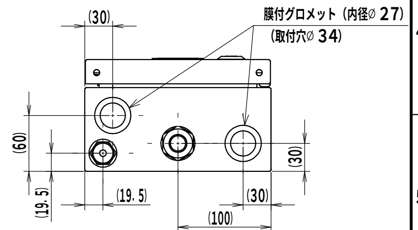
底面詳細図 (1:4)
