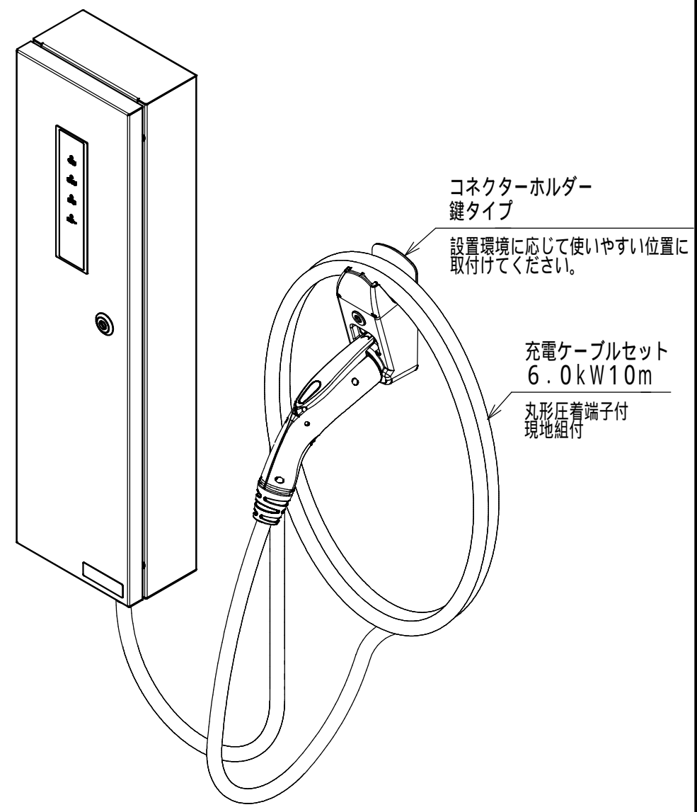
<取付例> 壁面取付
