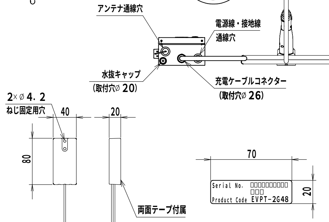
アンテナ詳細図 (1:4)
