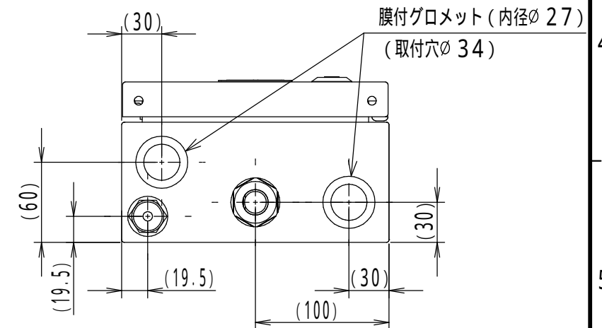
底面詳細図 (1:4)
