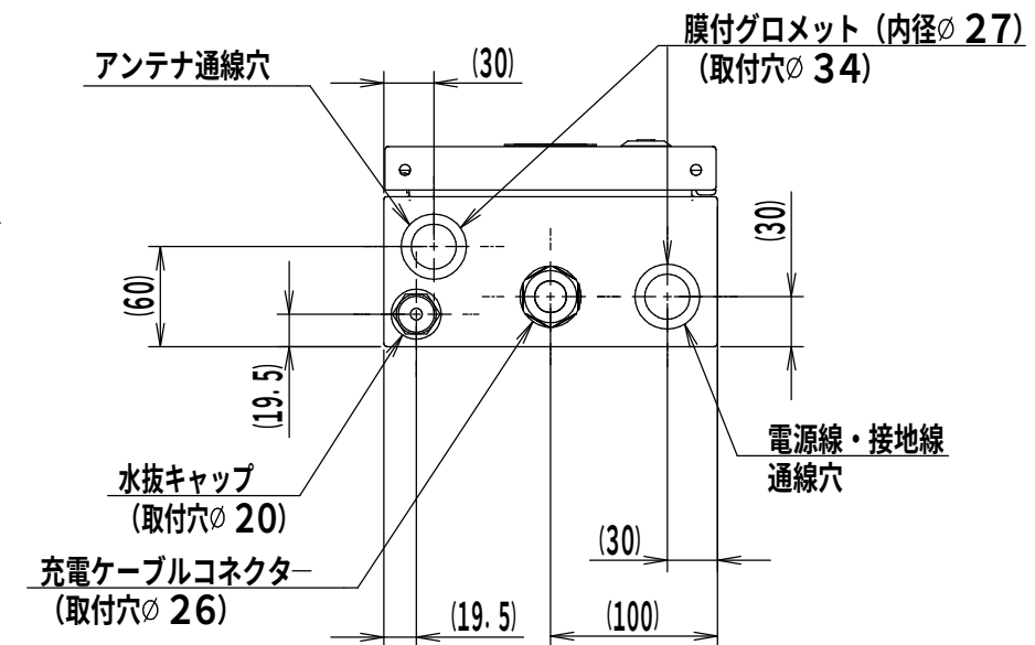
充電器本体の底面詳細図 (1:5)
