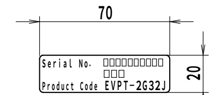
シリアルラベル詳細図 (1:2)
