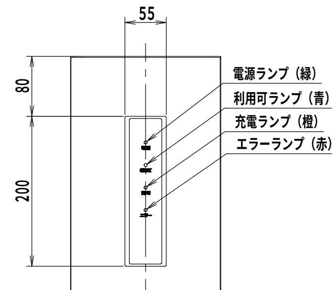
インフォメーションパネル詳細図 (1:5)
