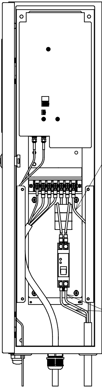
内部配線図 (1:5) 保護板 (下) を外した図
