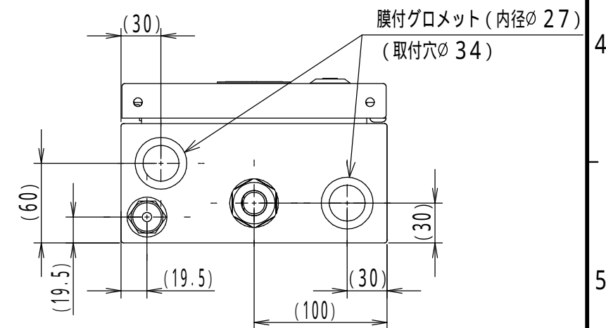
底面詳細図 (1:4)
