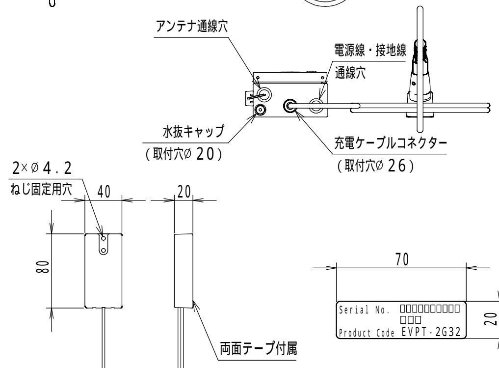
アンテナ詳細図 (1:4)
