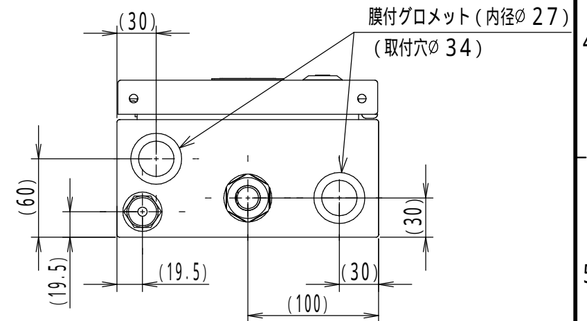
底面詳細図 (1:4)
