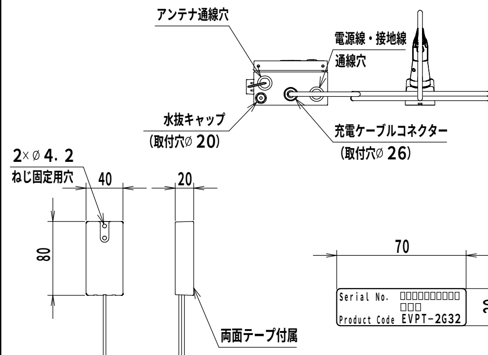
アンテナ詳細図 (1:4)
