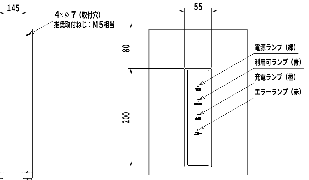
インフォメーションパネル詳細図 (1:4)
