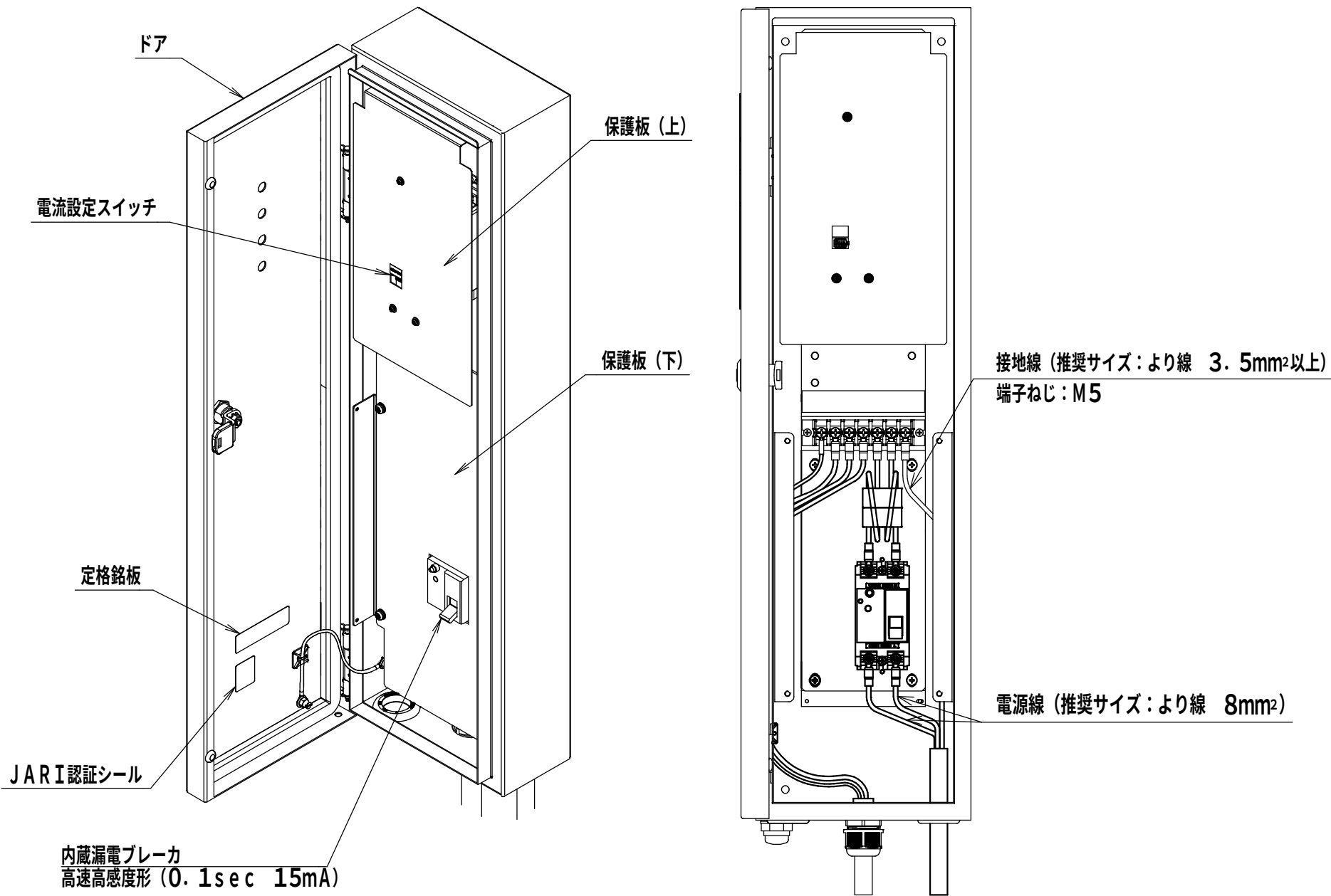
内部配線図 (1:5) 保護板 (下) を外した図
