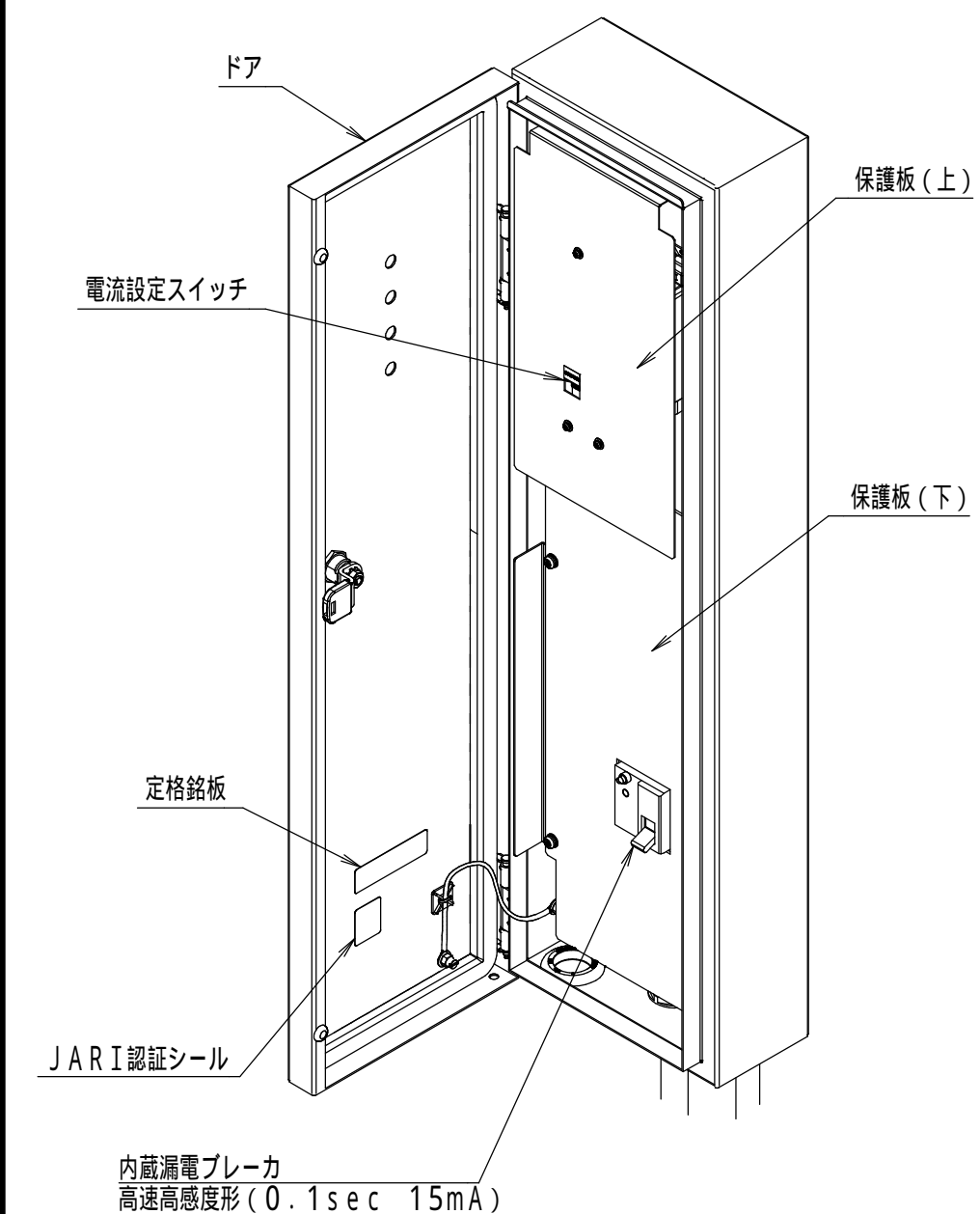
充電器内面図 ドアを開けた図
