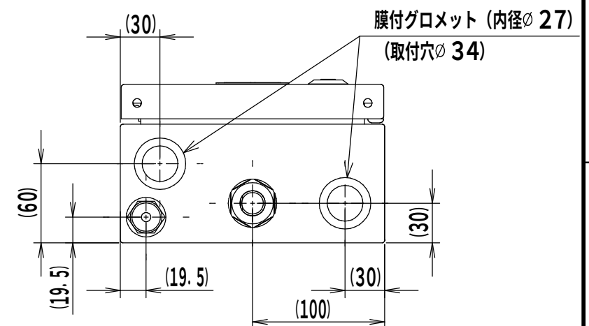
底面詳細図 (1:4)
