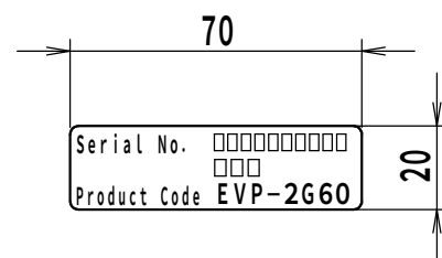
铭板シール詳細図 (1:2)
