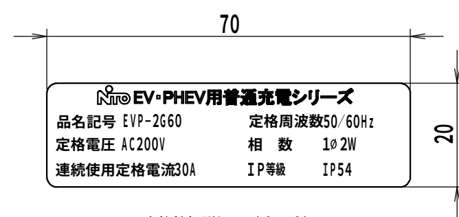
定格銘板詳細図 (1:1) (ドア裏貼付)
