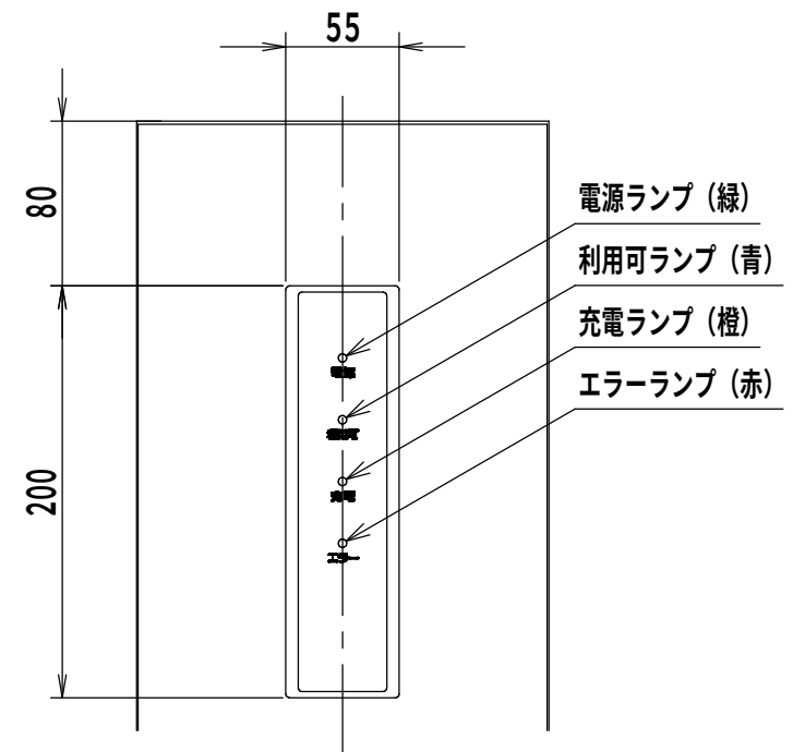
情報パネル詳細図 (1:4)
