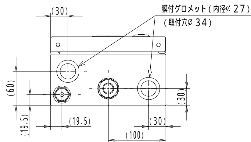
底面詳細図 (1:4)
