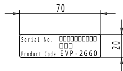
銘板シール詳細図 (1:2)
