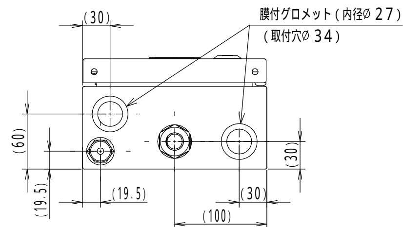
情報パネル詳細図 (1:4)
