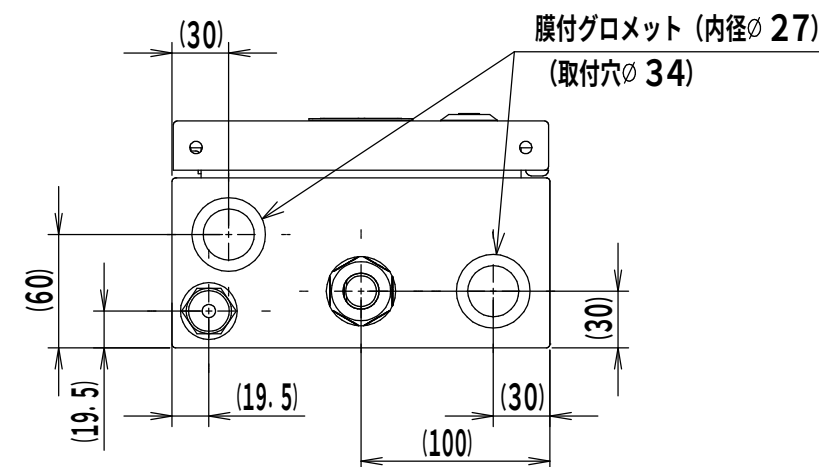
底面詳細図 (1:4)
