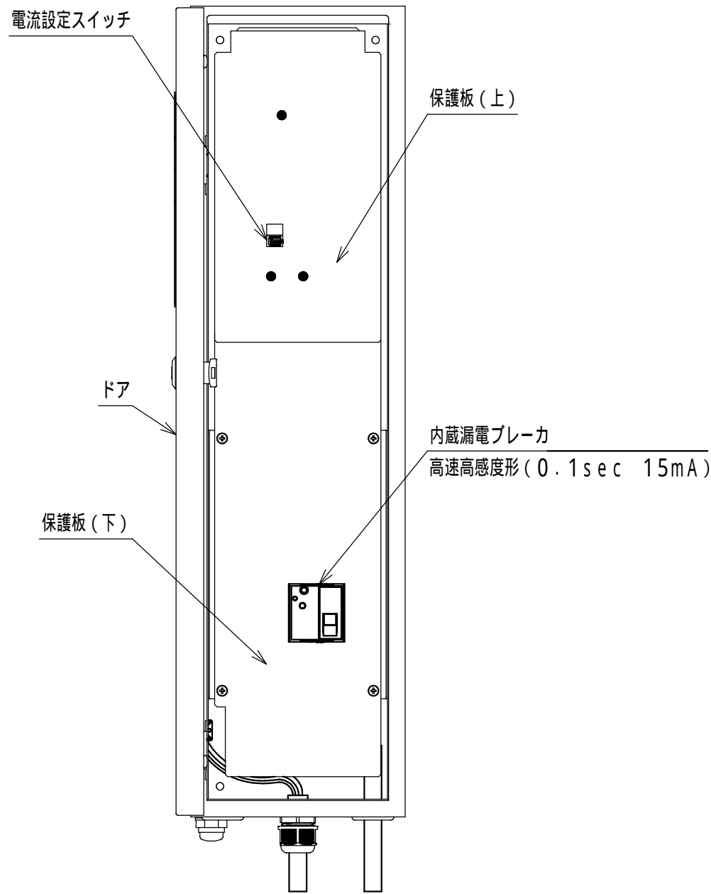
内面図（1：5） ドアを開けた図
