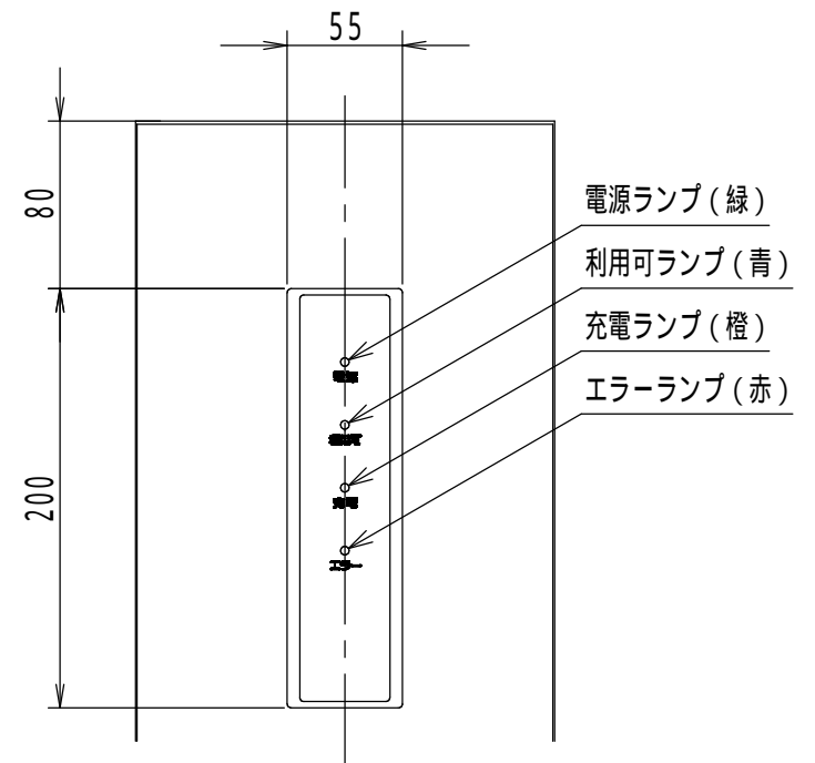
情報パネル詳細図 (1:4)
