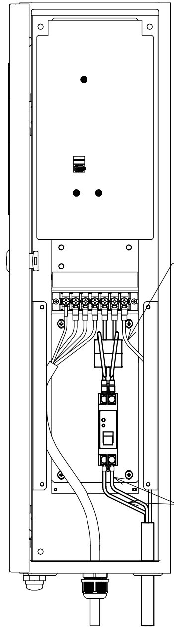
内部配線図 (1:5) 保護板(下)を外した図
