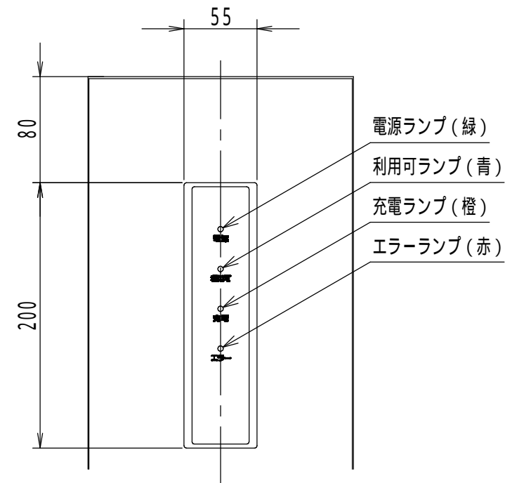
情報パネル詳細図 (1:4)
