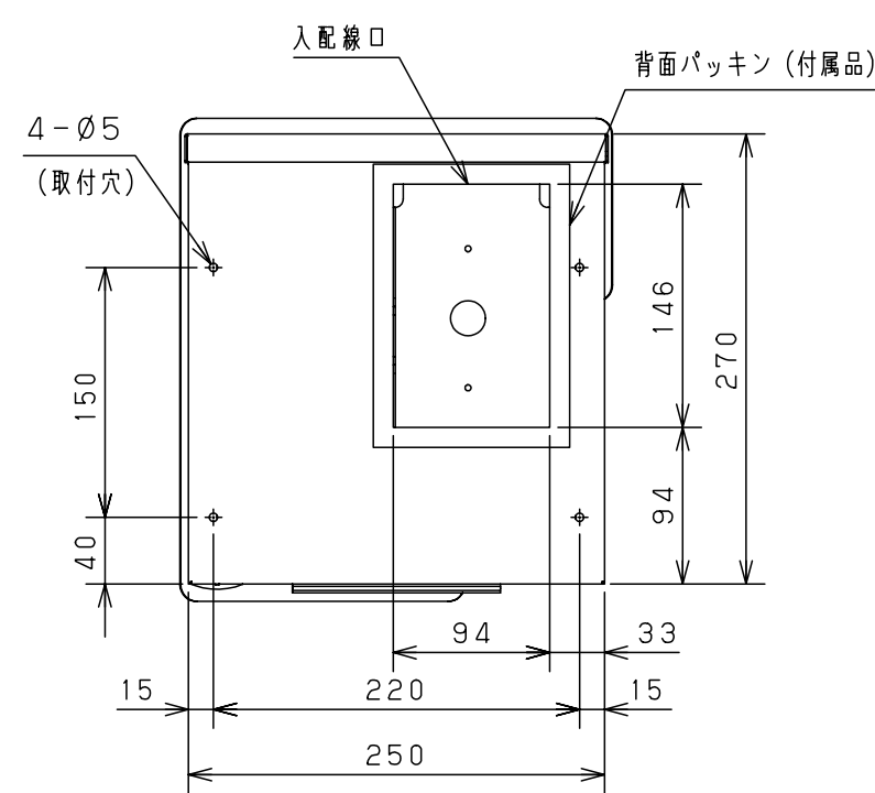
(背面図)
