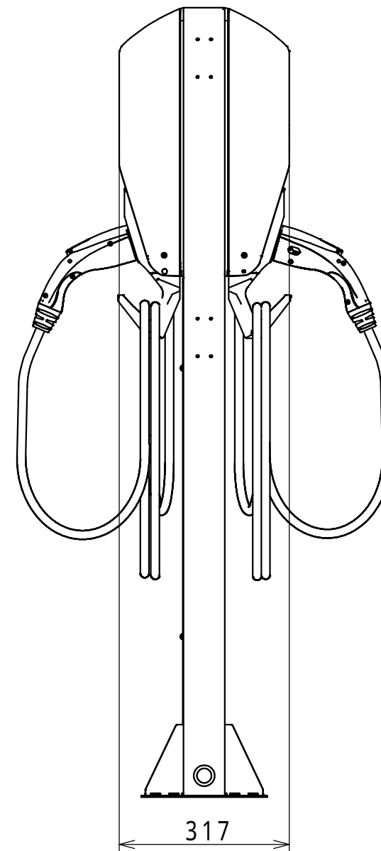
2台取付例
