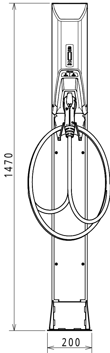
1台取付例
