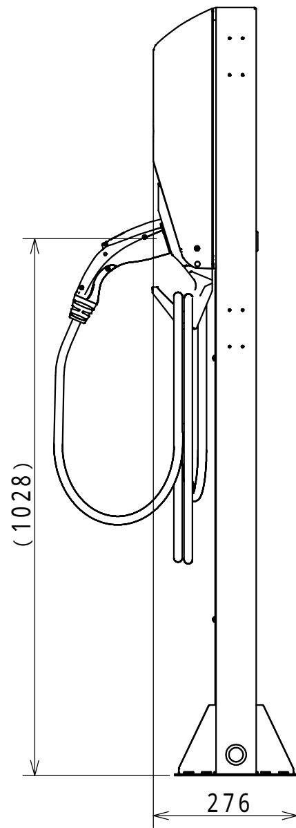
1台取付例
