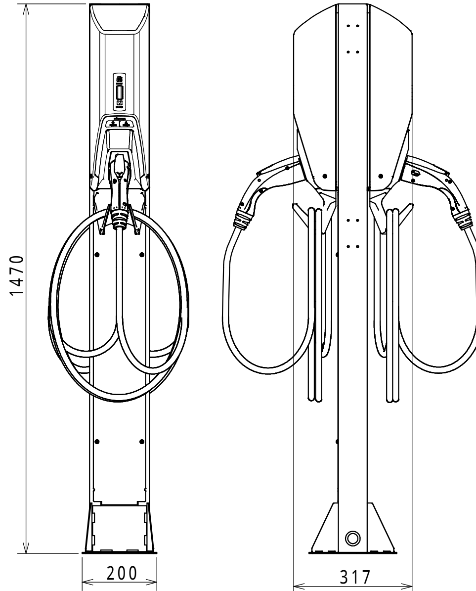
2台取付例
