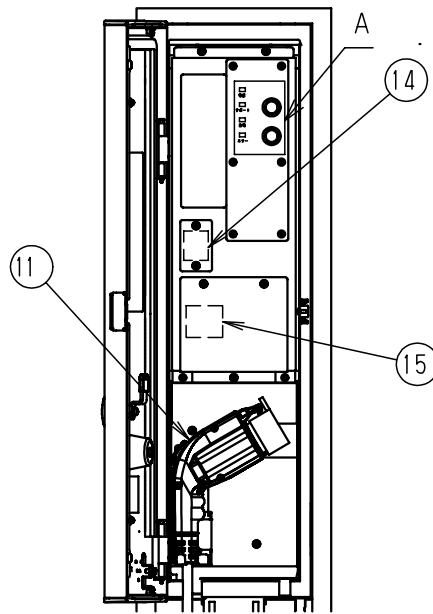
前面 内面図
