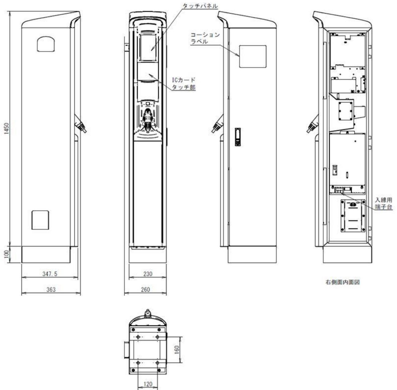
充電スタンド外形図
