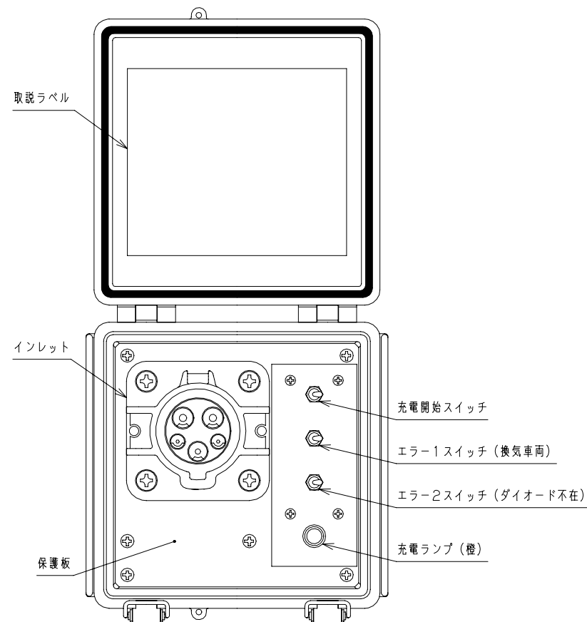
内観図
